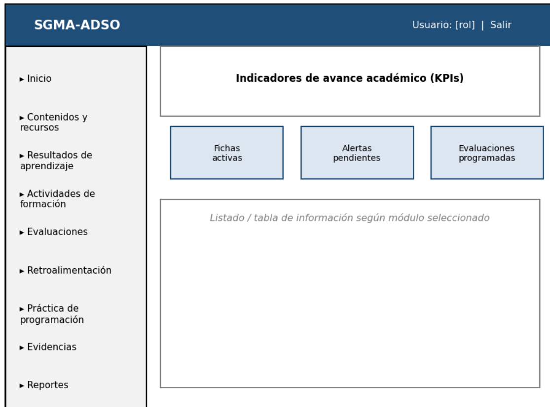
Figura. Wireframe - Pantalla principal (dashboard) con navegación por módulos.
