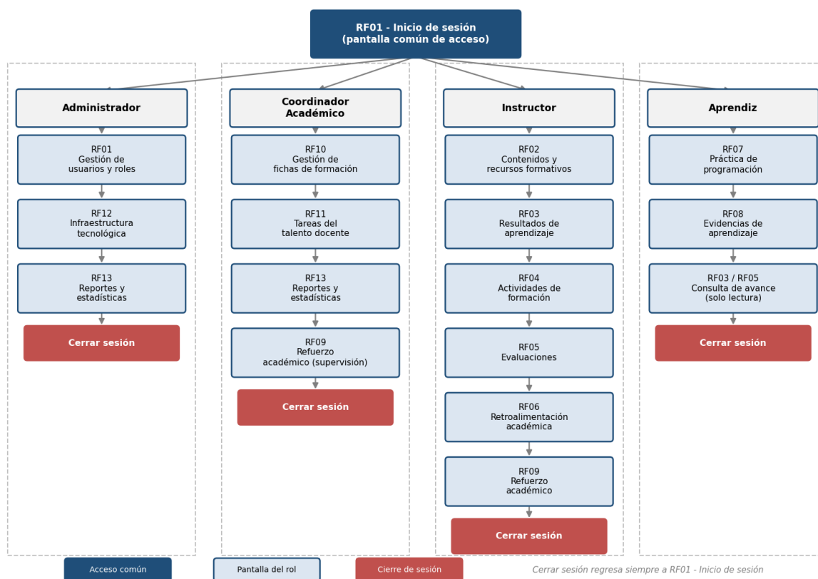
Figura. Mapa de navegación del sistema SGMA-ADSO, organizado por rol.
