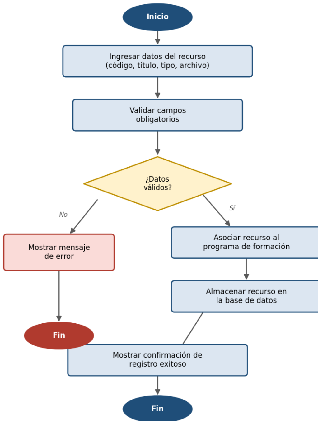
Figura. Diagrama de actividades - CU-RF02: Registro de recursos formativos.
