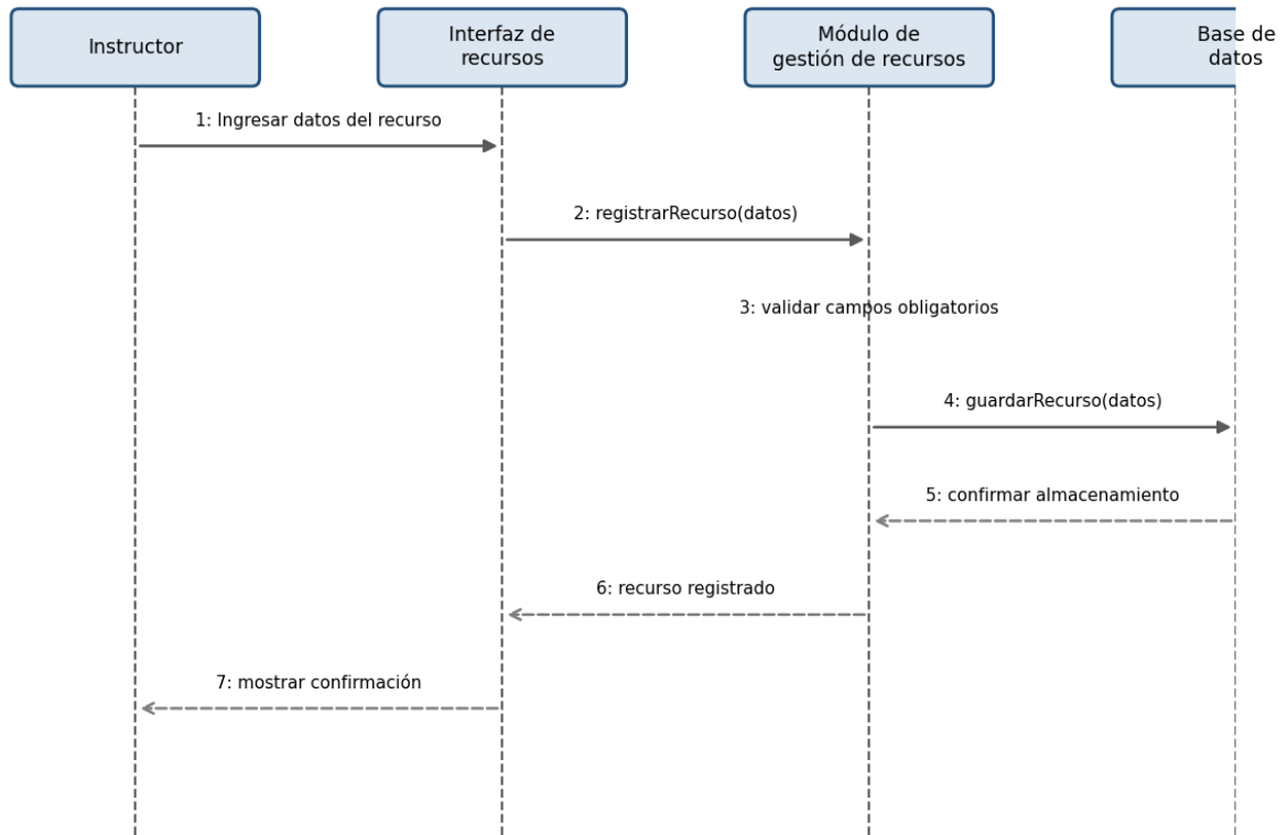
Figura. Diagrama de secuencia - CU-RF02: Registro de recursos formativos.
