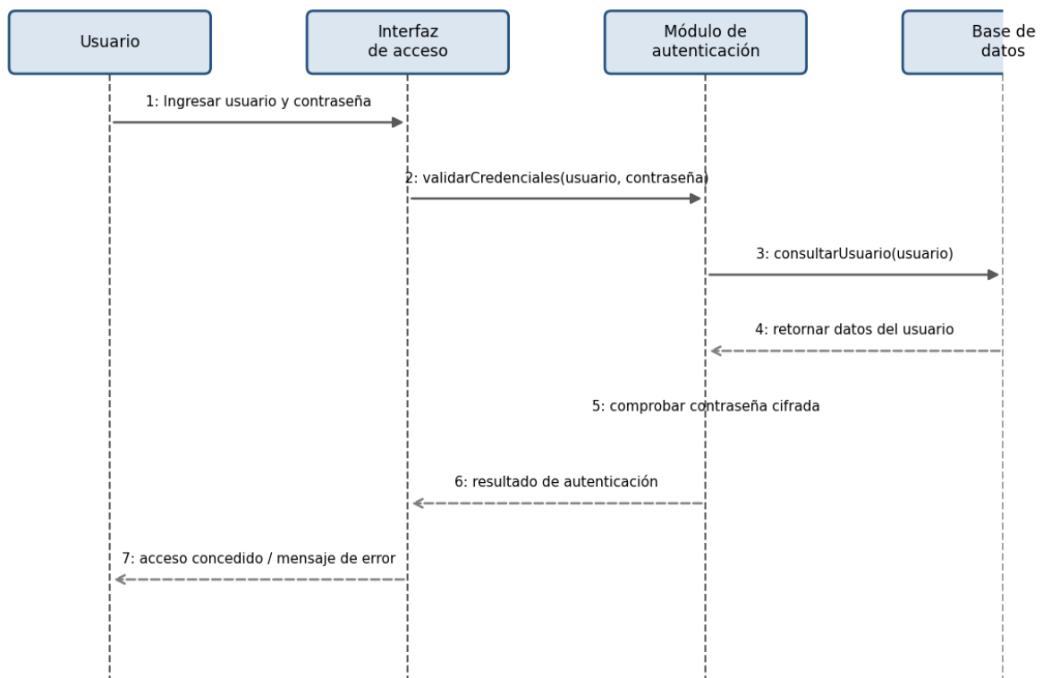
Figura. Diagrama de secuencia - CU-RF01: Inicio de sesión.
