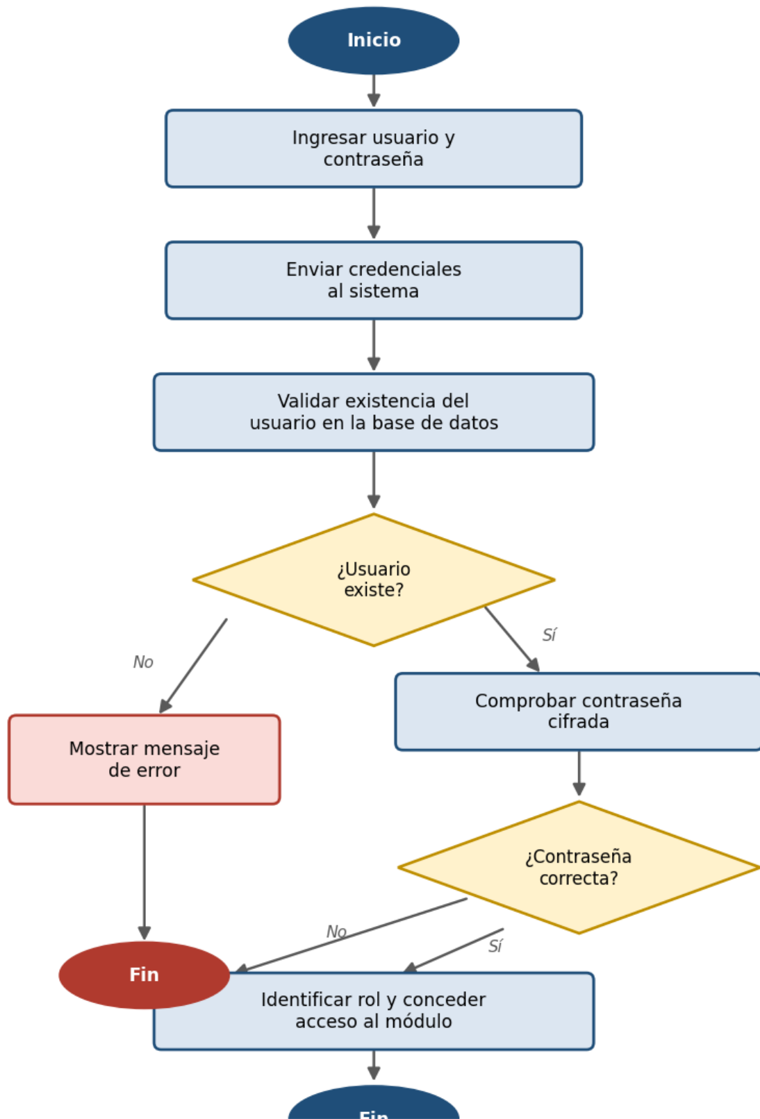
Figura. Diagrama de actividades - CU-RF01: Inicio de sesión.
